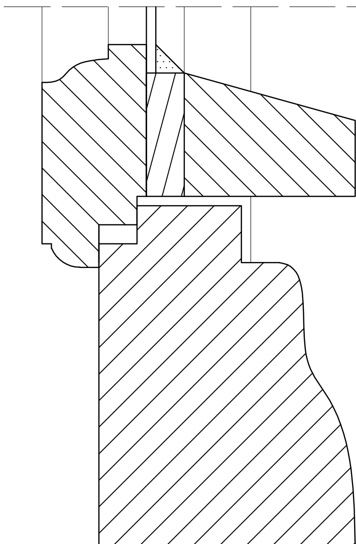
Okno Org. 1 - Detale powtarzające się we wszystkich oryginalnych stolarkach w obiekcie, skala 1:1
