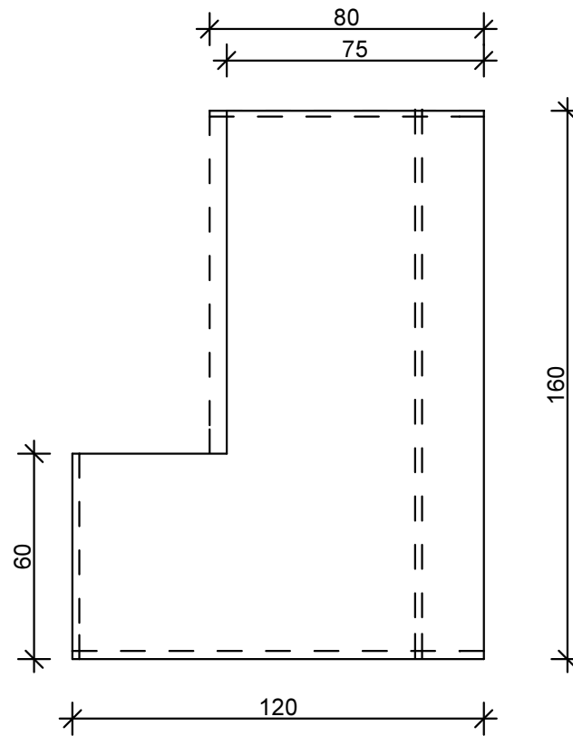
Bierko prostokątne narożne Rzut z góry
