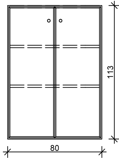
3 poziomy drzwi pelne
