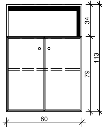
3 poziomy 1 poziom otwarty drzwi pelne
