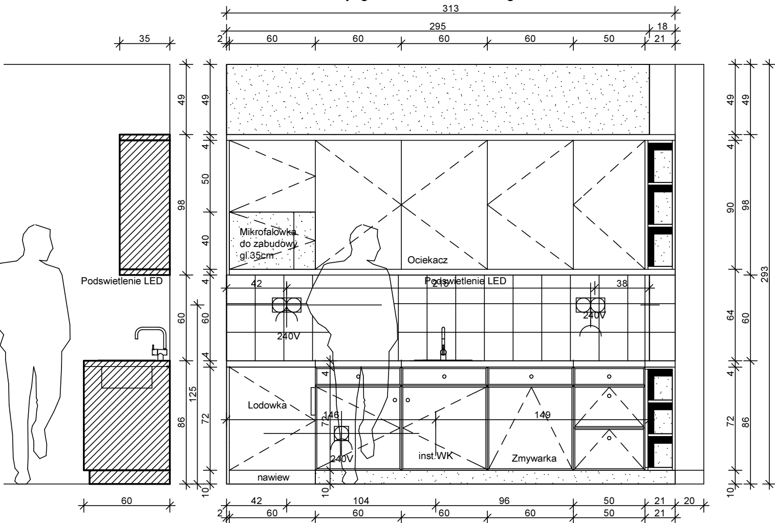
Przekroj
