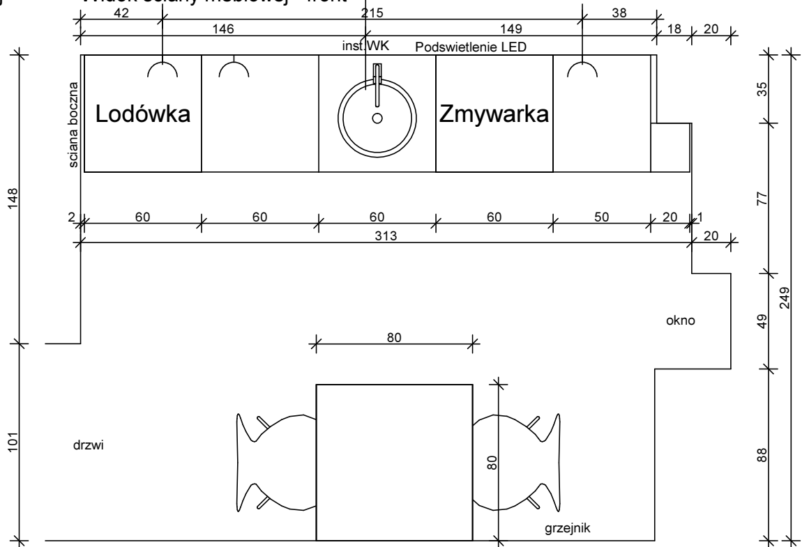
Rzut pomieszczenia.
