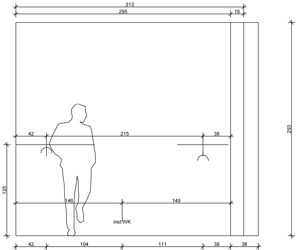
Widok sciany meblowej.
