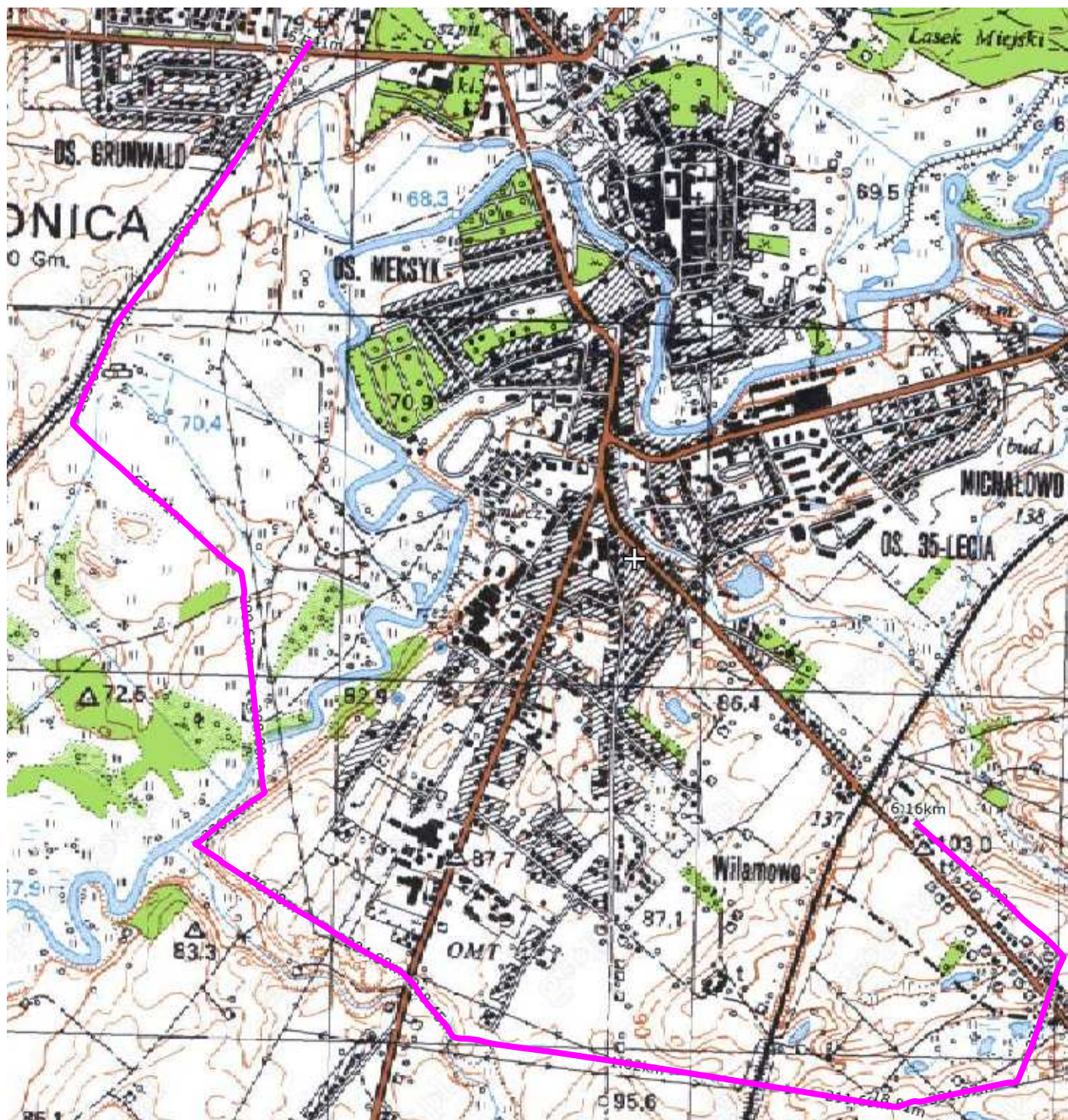
GPZ BRODNICA PODGÓRZ – GPZ BRODNICA GRUNWALD 6,2 km
